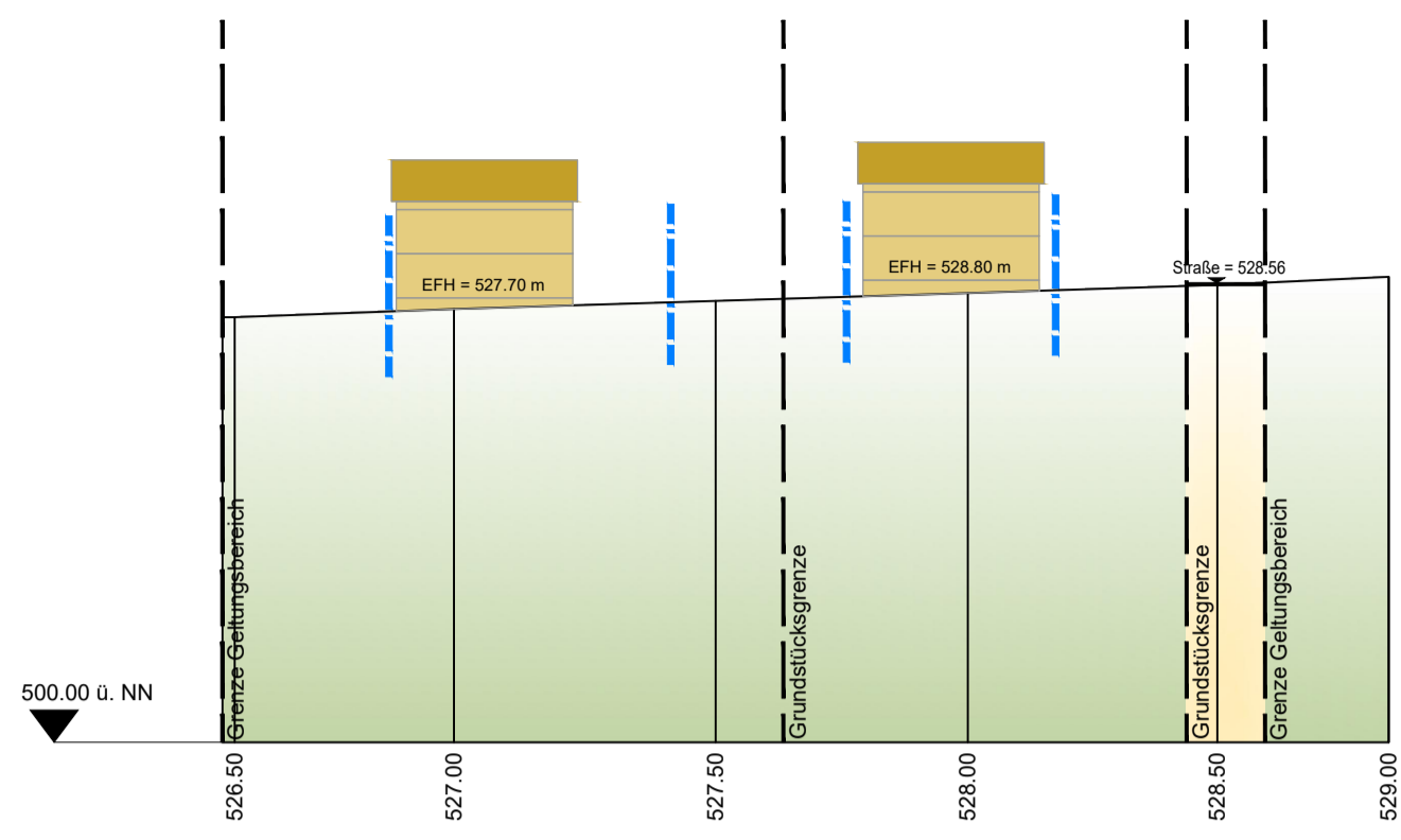
Schnitt B-B
