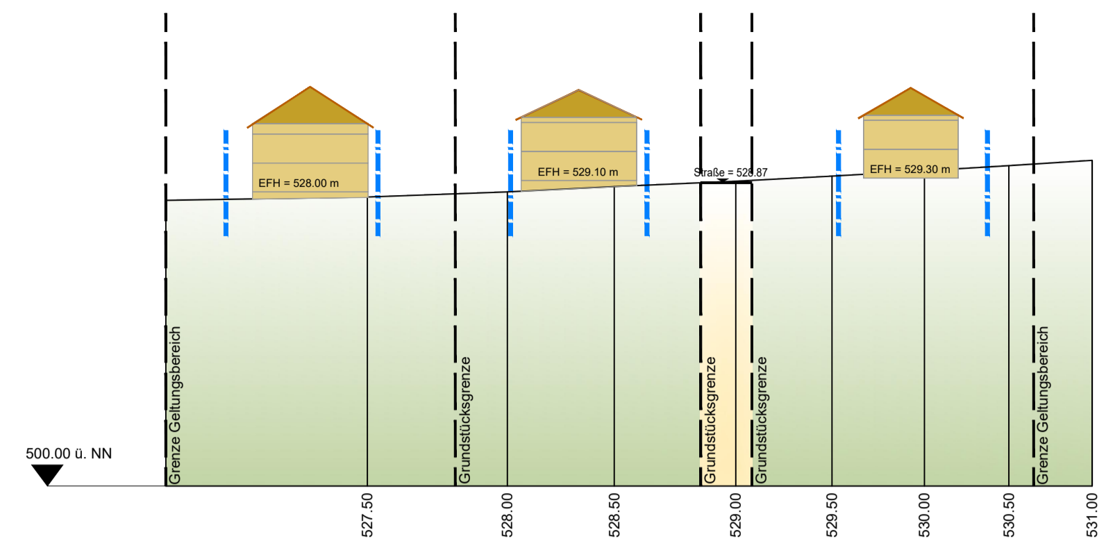
Schnitt F-F
