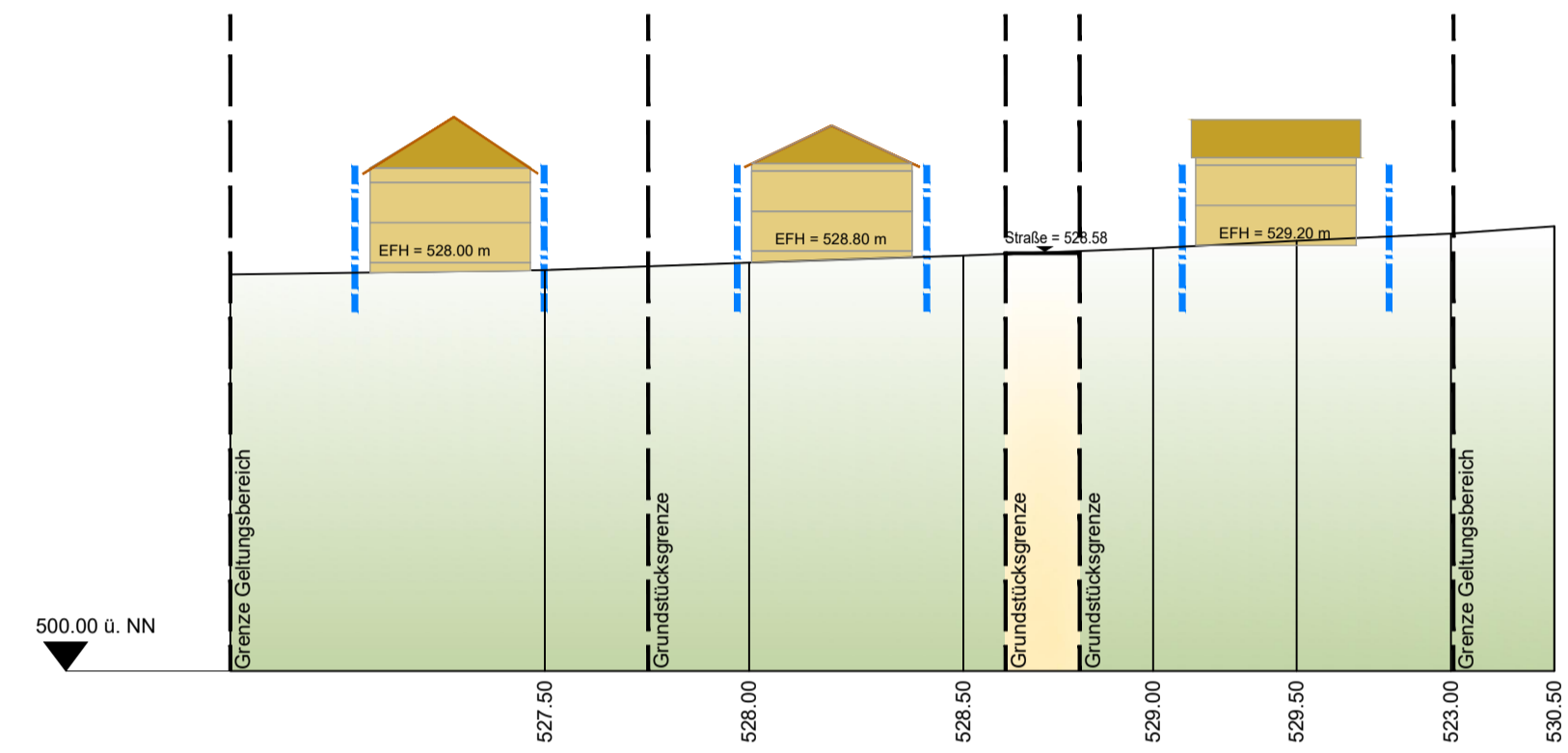
Schnitt G-G
