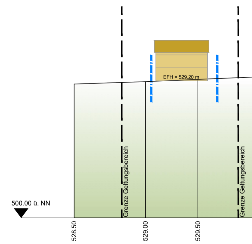
Schnitt G-G
