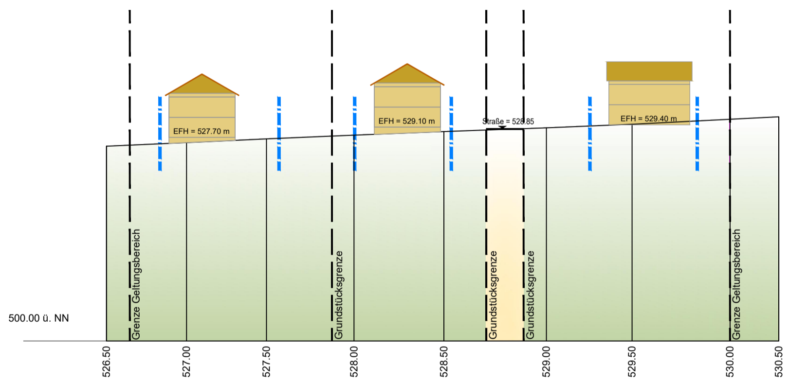
Schnitt D-D
