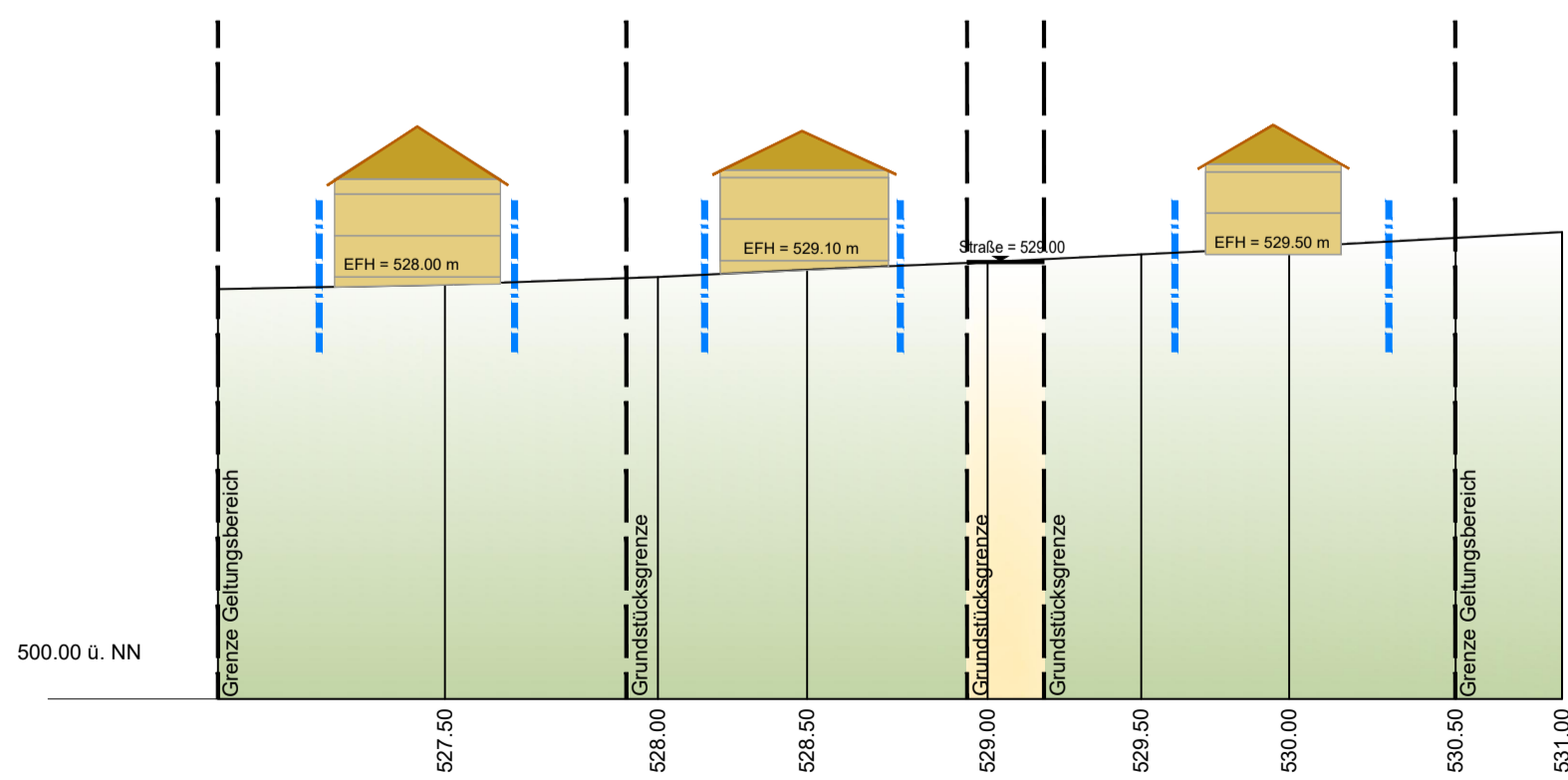
Schnitt D-D
