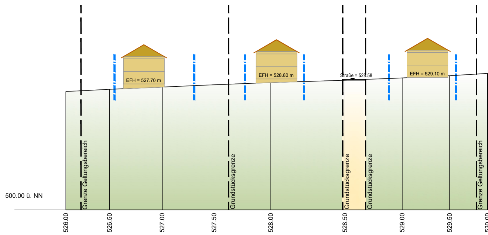
Schnitt C-C
